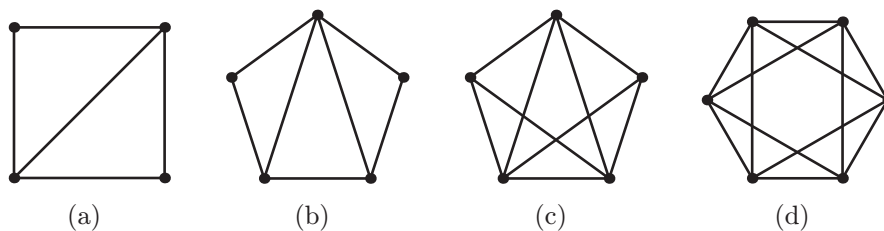
Obrázek 7.4: Určete počet koster.
