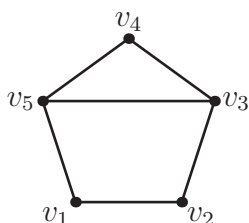
Obrázek 7.3: Graf z příkladu 7.12.
