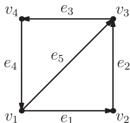
Obrázek 7.1: Orientovaný graf.
