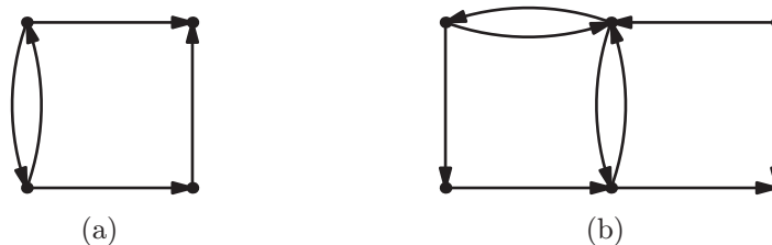
Obrázek 7.2: Určete incidenční matice.
